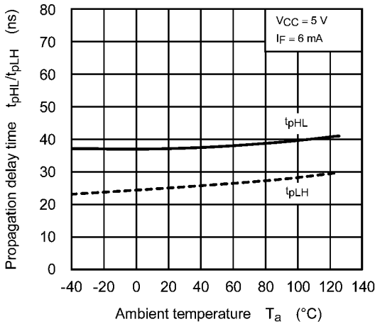
Fig. 12.2.11 t_{pHL}/t_{pLH} - T_a
