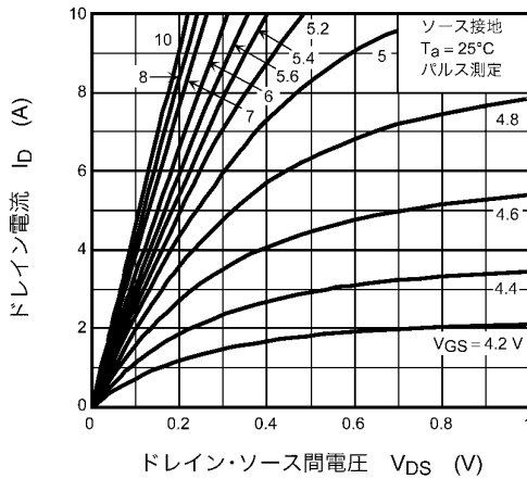
図 8.1 I_D - V_{DS}
