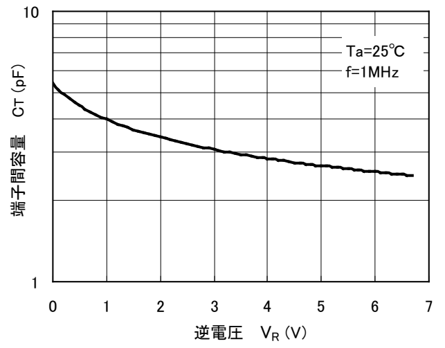
C_T - V_R
