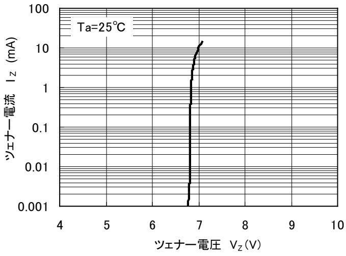
I_Z - V_Z
