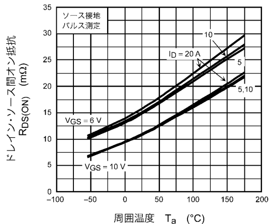
図 8.6 R_{DS(ON)} - T_a
