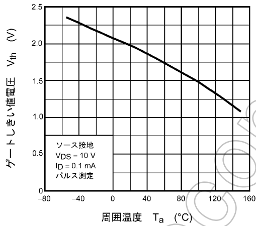
図 8.2.9 V_{th} - T_a
