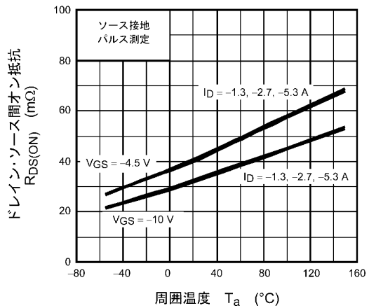
図 8.1.6 R_{DS(ON)} - T_a
