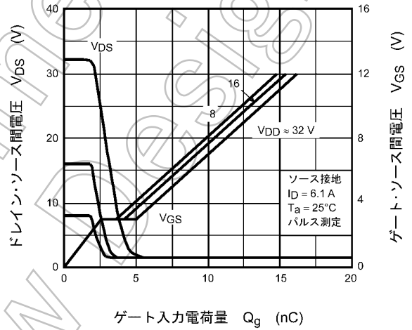
図 8.2.10 ダイナミック入出力特性
