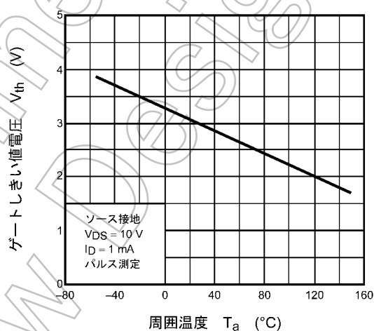
図 8.10 V_{th} - T_a
