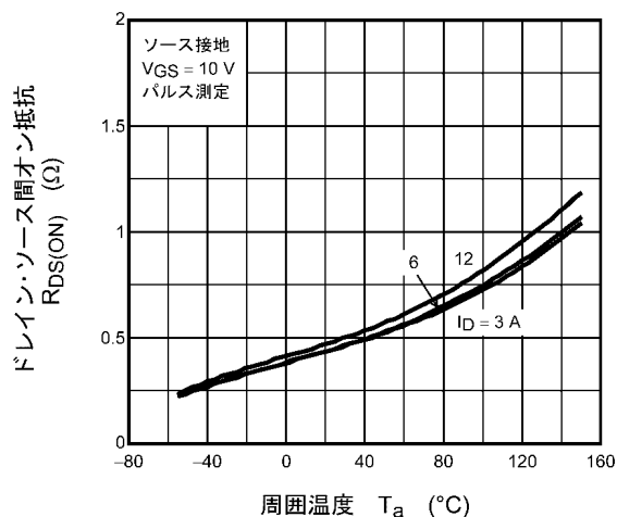
図 8.7 R_{DS(ON)} - T_a
