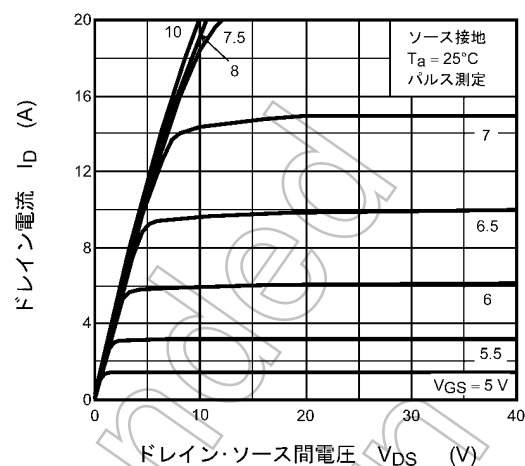
図 8.2 I_D - V_{DS}
