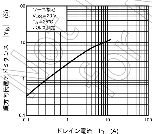
図 8.5 |Y_{fs}| - I_D
