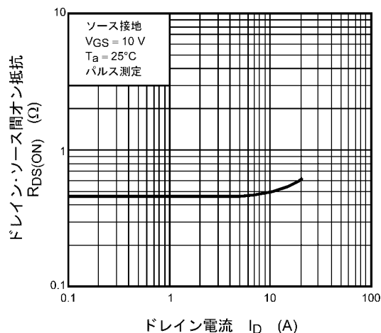
図 8.6 R_{DS(on)} - I_D
