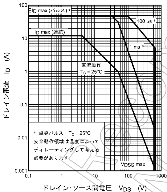
図 8.14 安全動作領域 (最大値 (保証値))
