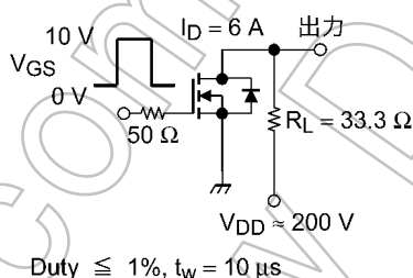
図 6.2.1 スwitchング時間の測定回路例
