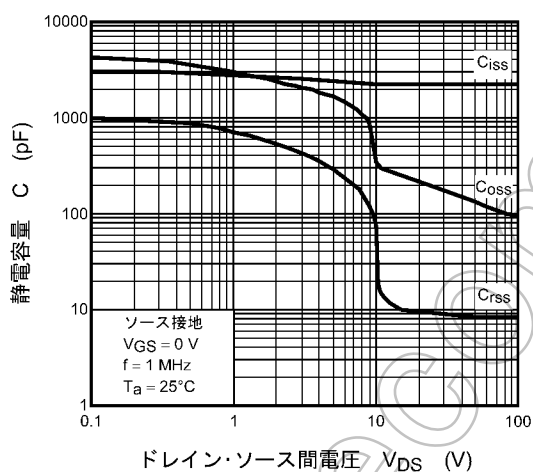
図 8.9 C - V_{DS}
