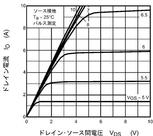
図 8.1 I_D - V_{DS}
