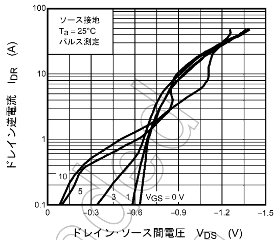
図 8.8 I_{DR} - V_{DS}
