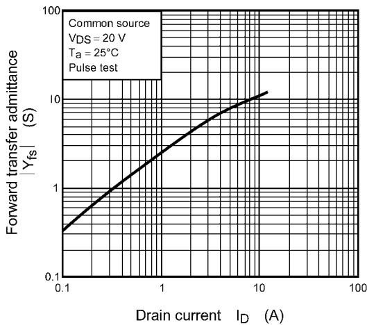
Fig. 8.5 |Y_{fs}| - I_D
