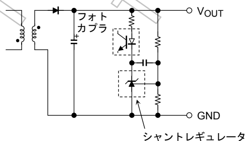
スイッチング電源の誤差増幅回路
