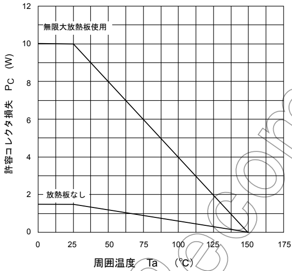
P_c-T_a
