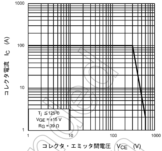
図 8.12 逆バイアス安全動作領域 (最大値 (保証値))
