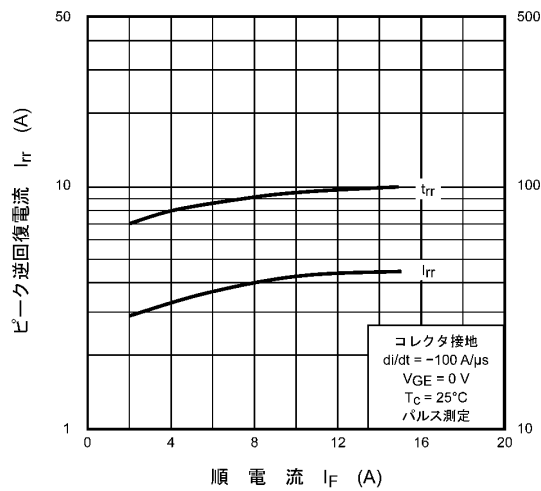
図 8.15 I rr , t rr - I F
