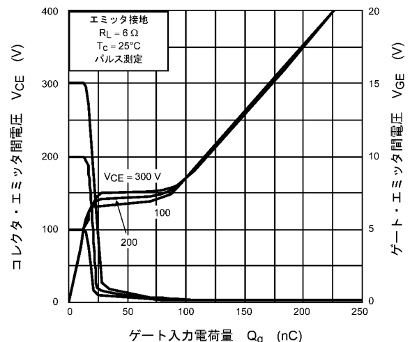
図 8.6 V_{CE}, V_{GE} - Q_g
