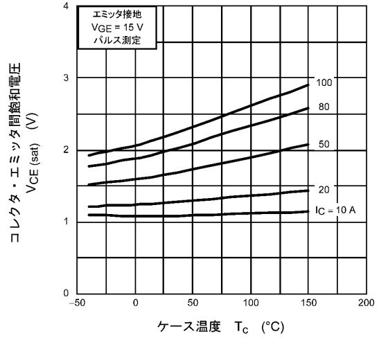
図 8.4 V_{ce(sat)} - T_c
