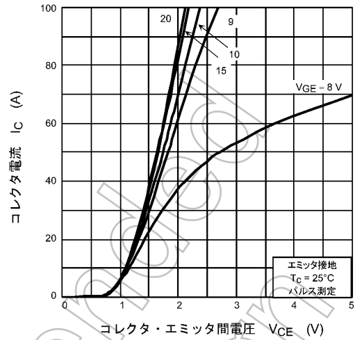
図 8.2 I_c - V_{CE}
