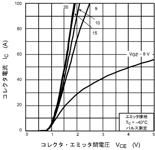
図 8.1 I_c - V_{CE}
