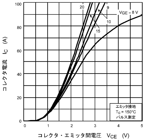
図 8.3 I_c - V_{ce}
