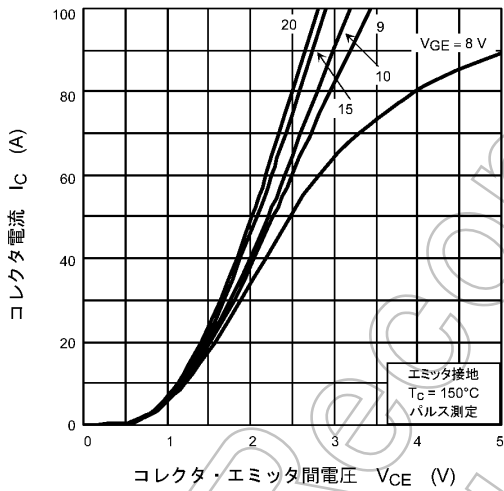
図 8.3 I_c - V_{CE}
