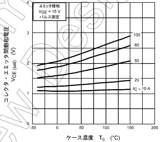
図 8.4 V_{CE}(\text{sat}) - T_c
