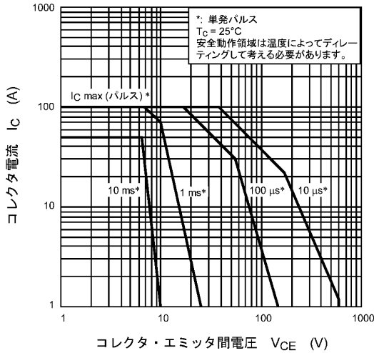
図 8.11 安全動作領域 (最大値 (保証値))
