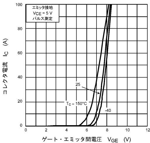
図 8.5 I_c - V_{ge}
