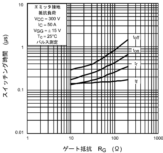
図 8.9 スイッチング時間 - R G
