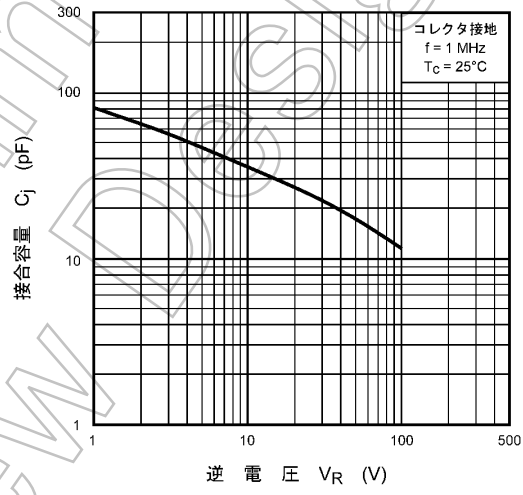
図 8.14 C j - V R
