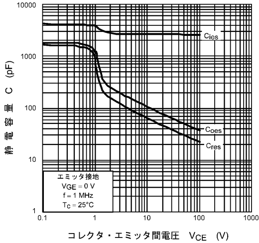
図 8.7 C-V CE
