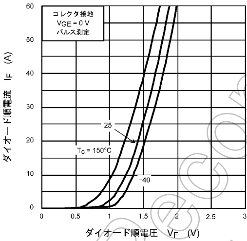
図 8.13 I F - V F
