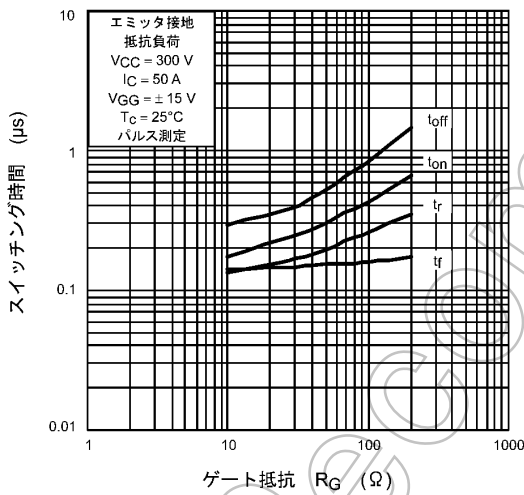
図 8.9 スイッチング時間 - R G
