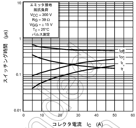
図 8.8 スイッチング時間 - I C
