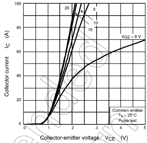
Fig. 8.2 I_C - V_{CE}
