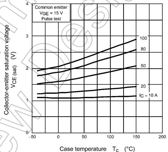
Fig. 8.4 V_{CE(sat)} - T_C
