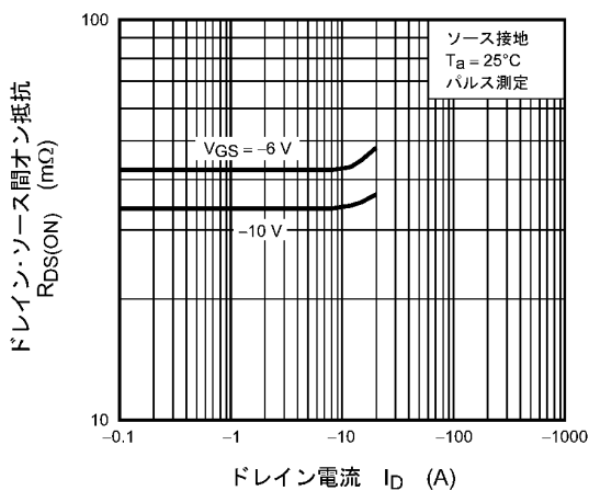
図 8.5 R_{DS(ON)} - I_D
