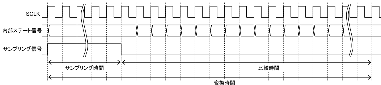
図 3.6 変換タイミング例
