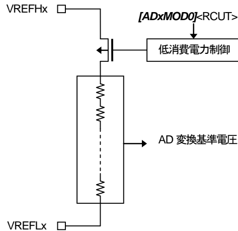
図 3.5 アナログ基準電圧回路構成
