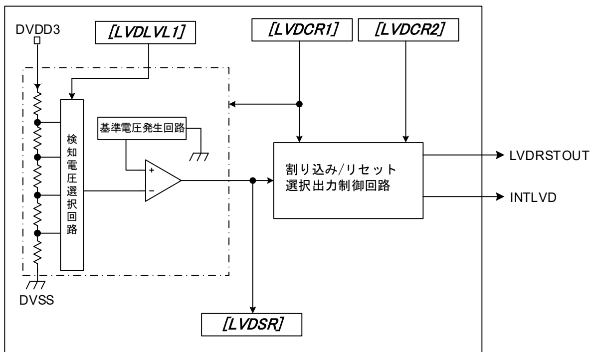
図 2.1 LVDのブロック図
