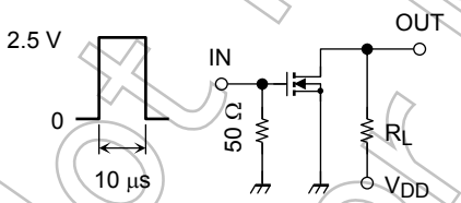
(a) 測定回路
