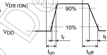
(c) 出力波形
