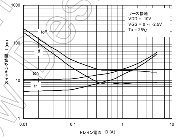
t - ID
